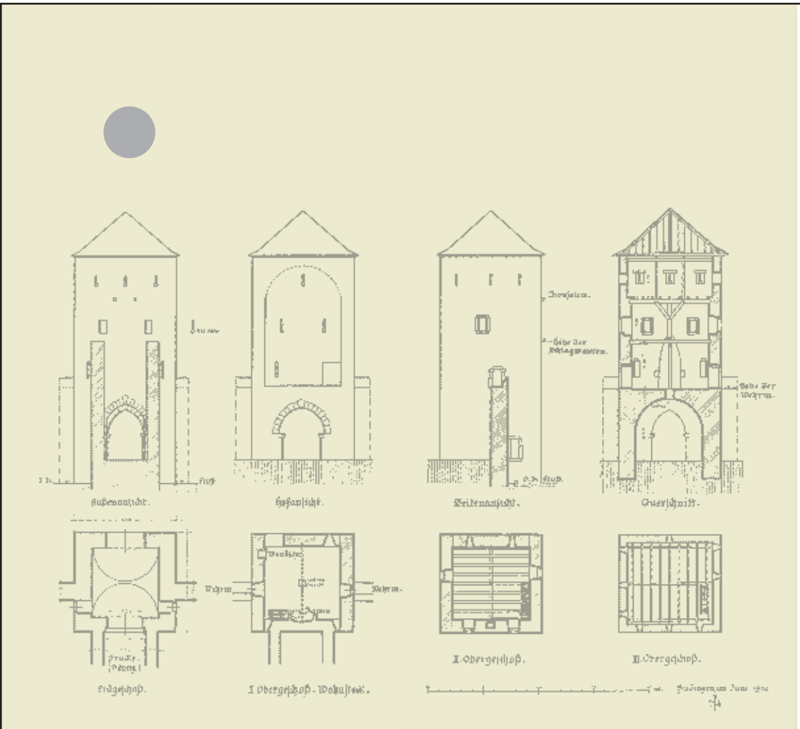
Schnitte und Grundrisse des Torturms
